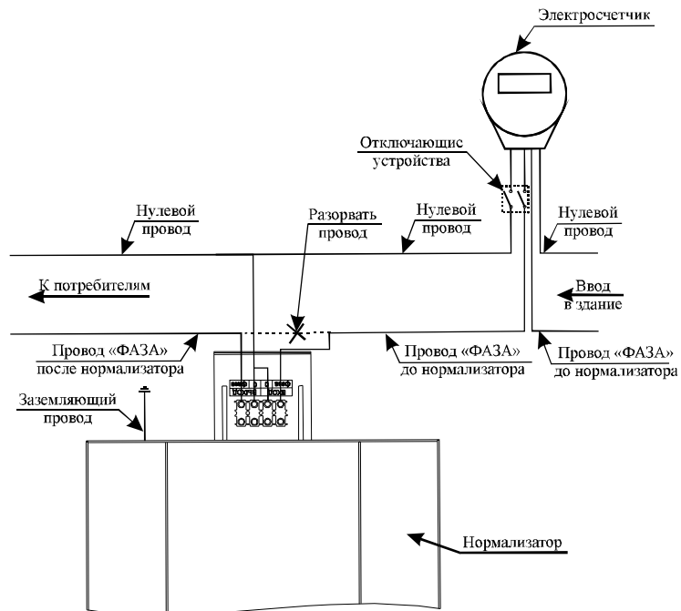
Рисунок 6. Подключение нормализатора, не разрывая нулевой провод.
