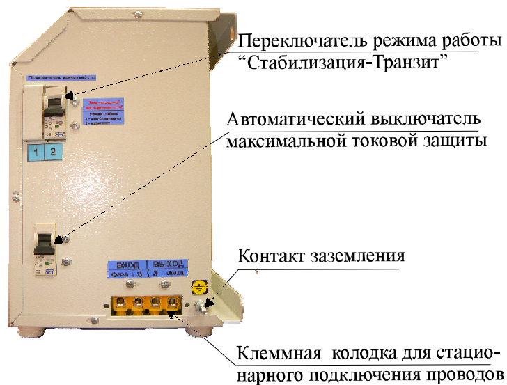
Рисунок 2. Общий вид нормализатора серии BREEZE
