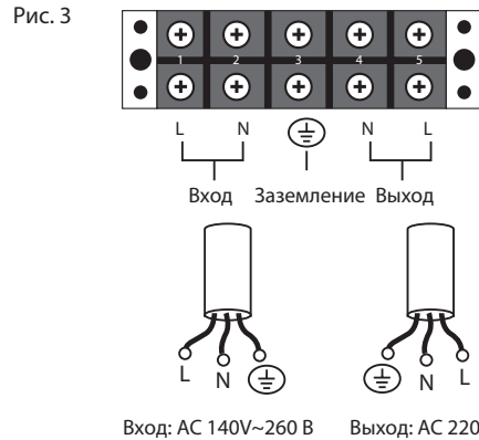
Вход: AC 140V~260 В Выход: AC 220 В
