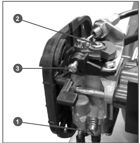
Рис. 15 Расположение винтов карбюратора 1. Винт «L» 2. Винт «H» 3. Винт «T»
