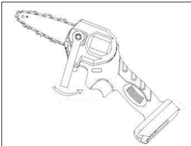
Рис. 1. Откручивание крепежного винта шины
