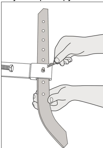
Рис.13. Установка сошника
