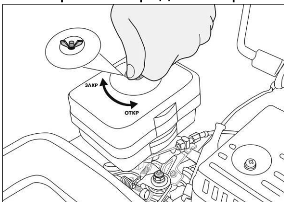
Рис. 19. Открытие крышки корпуса воздушного фильтра
