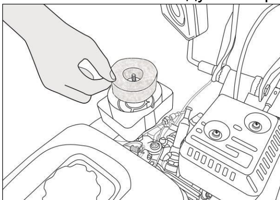
Рис. 36. Установка воздушного фильтра
