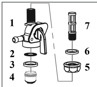
Рис. 19 Устройство топливного крана
