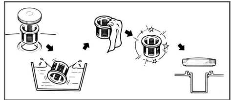
Рис. 18 Обслуживание фильтра топливного бака
