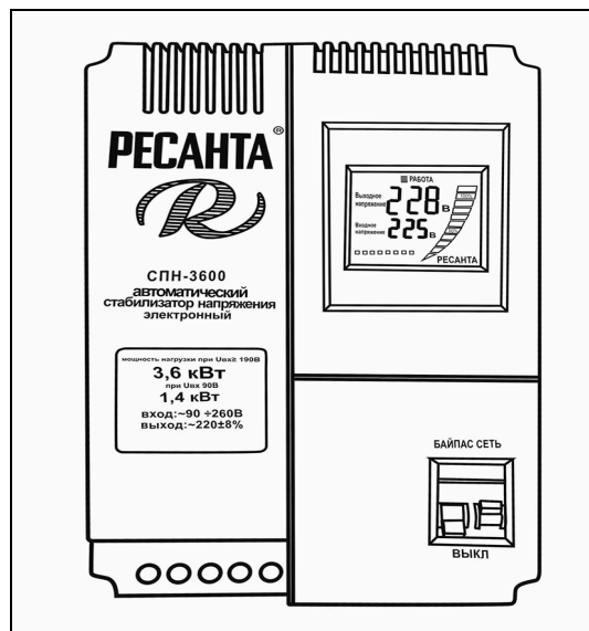
Рис.6. Показания дисплея после подключения нагрузки моделей СПН-3600 и более
