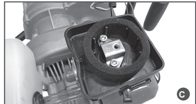
Рис. 11 Обслуживание воздушного фильтра
