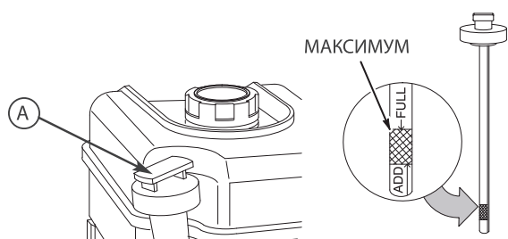
Проверка уровня масла
