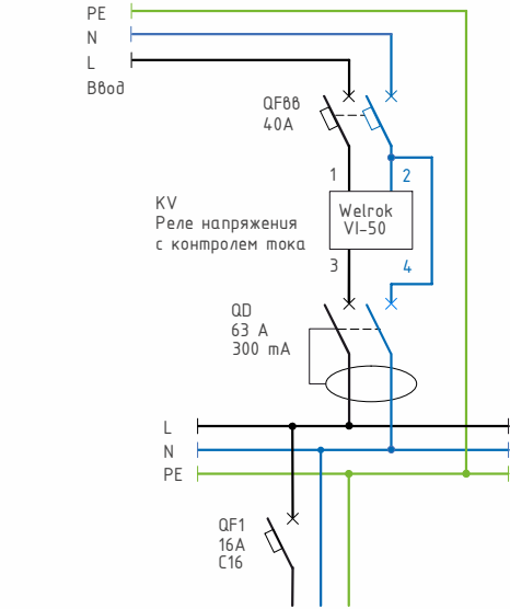
Схема 1. Вариант электрической схемы
