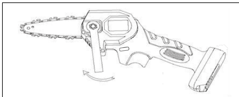
Рис. 3. Фиксация шины прижимной крышкой
