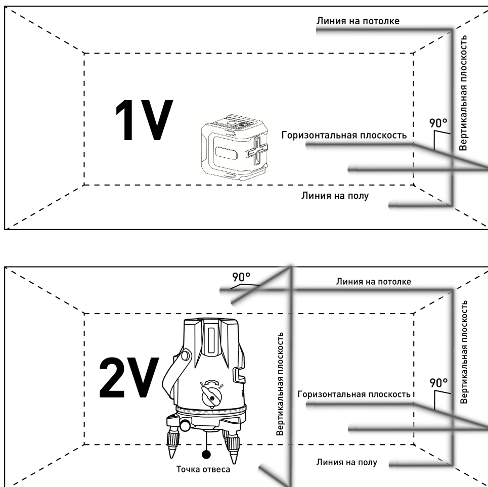
Рис.2 Лазерные плоскости (ПЛ-2, ПЛ-2 Green, ПЛ-2ШК, ПЛ-2ШК Green сверху; ПЛ-3, ПЛ-3 Green, ПЛ-3ШК снизу).
