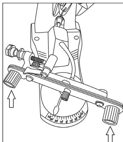
Рис.14 Перемещение цепи
