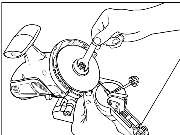
Рис.18 снятие круга
