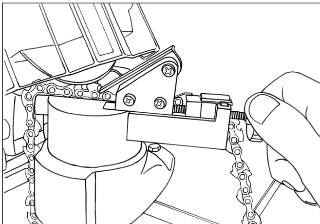
Рис.9 Регулировка зуба
