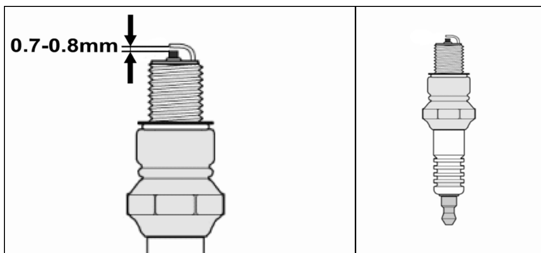
Рис. 25. Свеча зажигания
