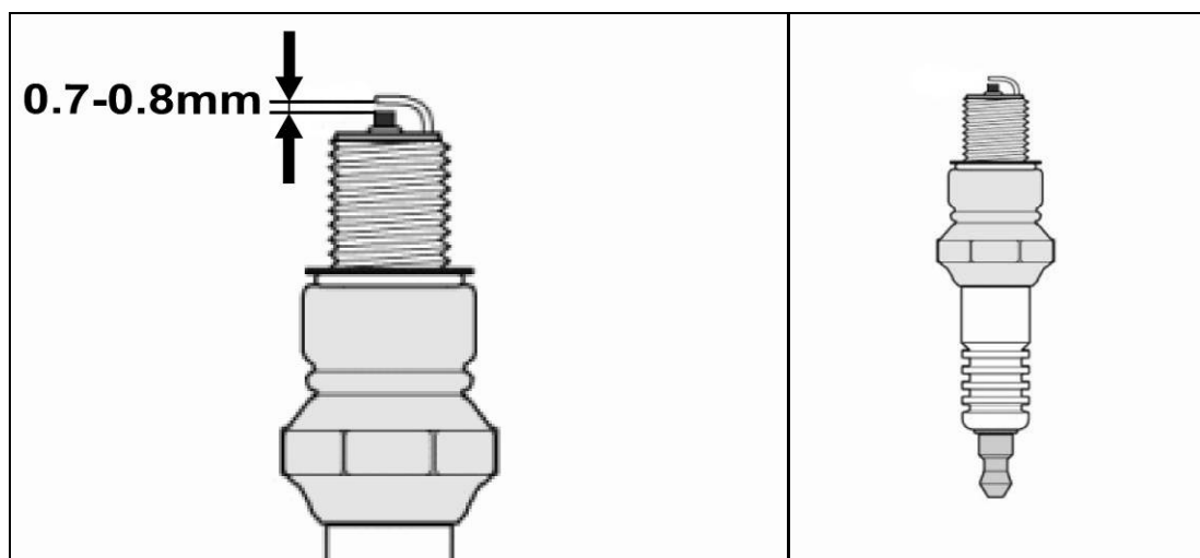
Рис. 25. Свеча зажигания
