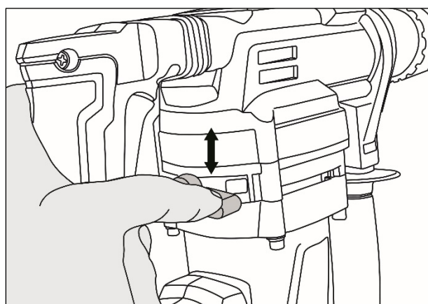
Рис. 10. Переключатель 1
