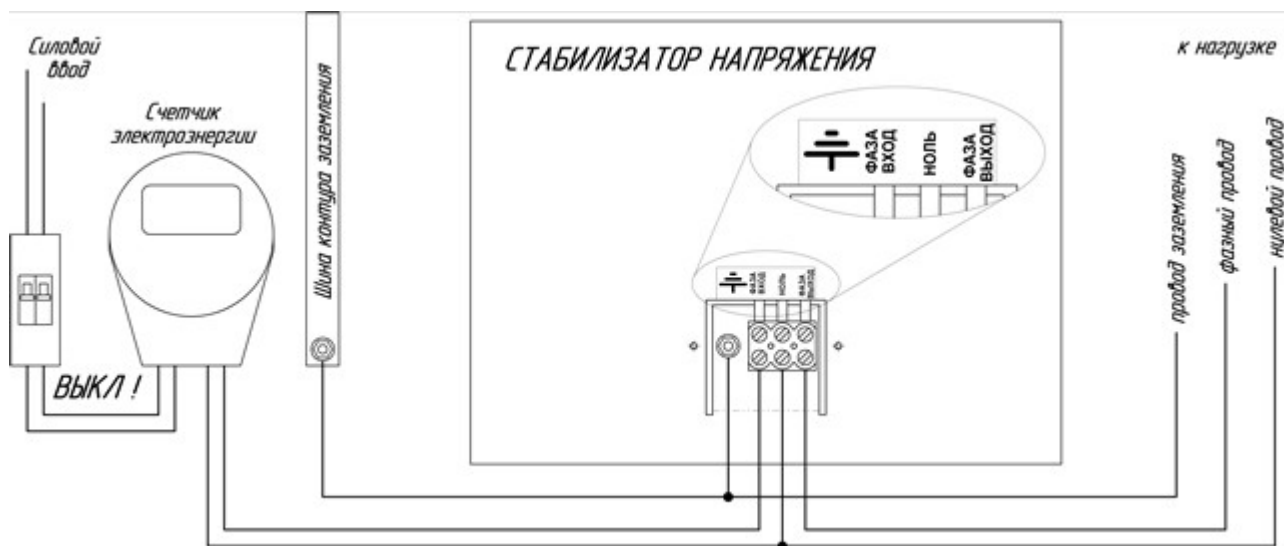
Рисунок 2. Рекомендуемая схема подключения стабилизатора к сети.
