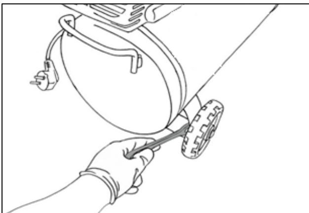
Рис. 5. Установка колес
