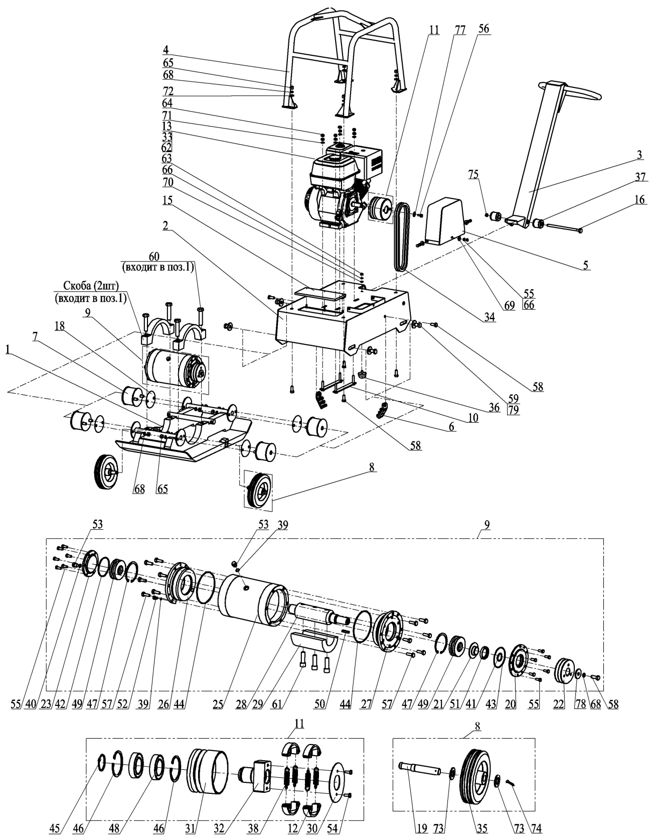
Рисунок 9 – Компоновка виброплиты
