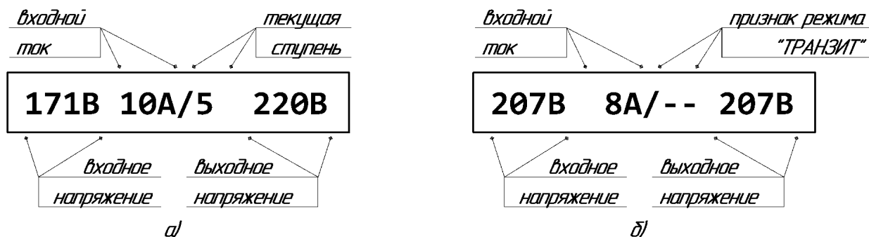
Рисунок 2. Примеры изображений на индикаторе стабилизатора («нулевой экран») а) в режиме «Стабилизация»; б) в режиме «Транзит».
