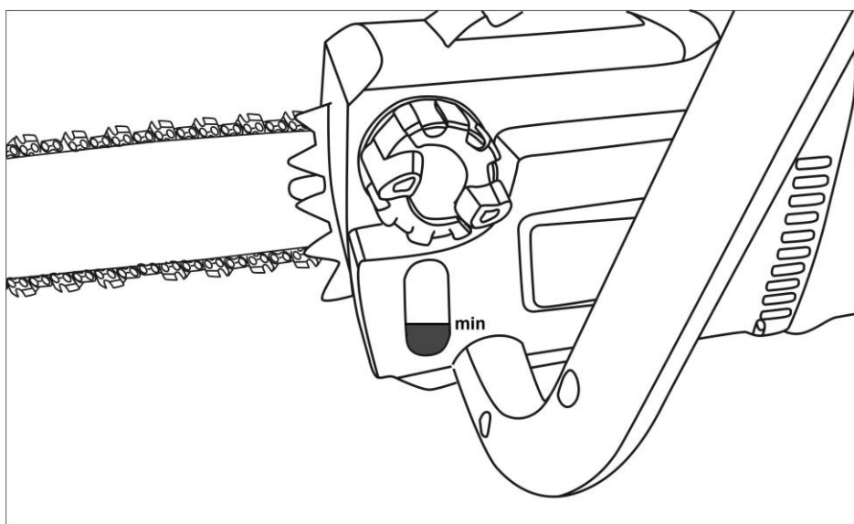
Рис. 10. Смотровое окно масляного бака
