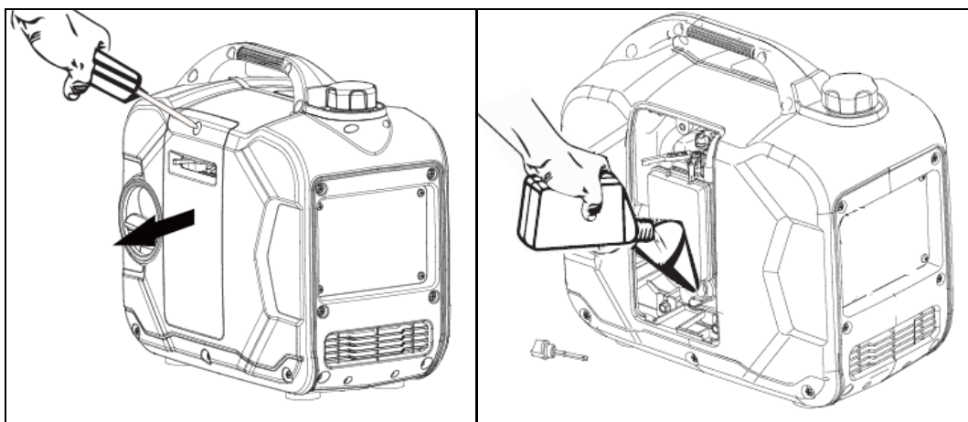
Рис. 3. Снятие сервисной панели кожуха генератора
