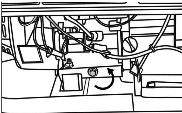
Рис. 10. Слив масла
