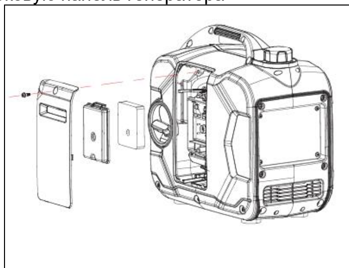
Рис. 15. Снятие сервисной панели кожуха генератора
