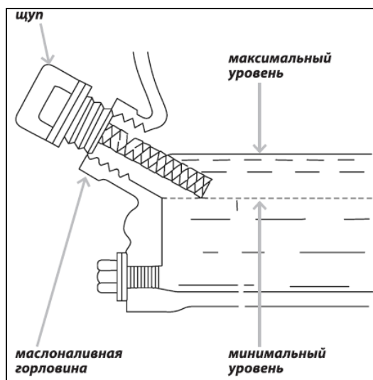
Рис. 4. Уровень масла
