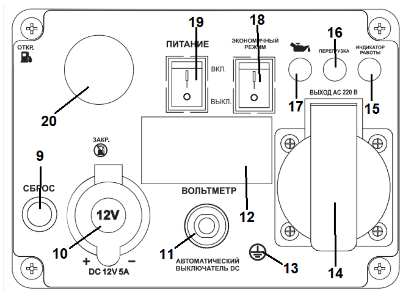
Рис. 2. Панель управления
