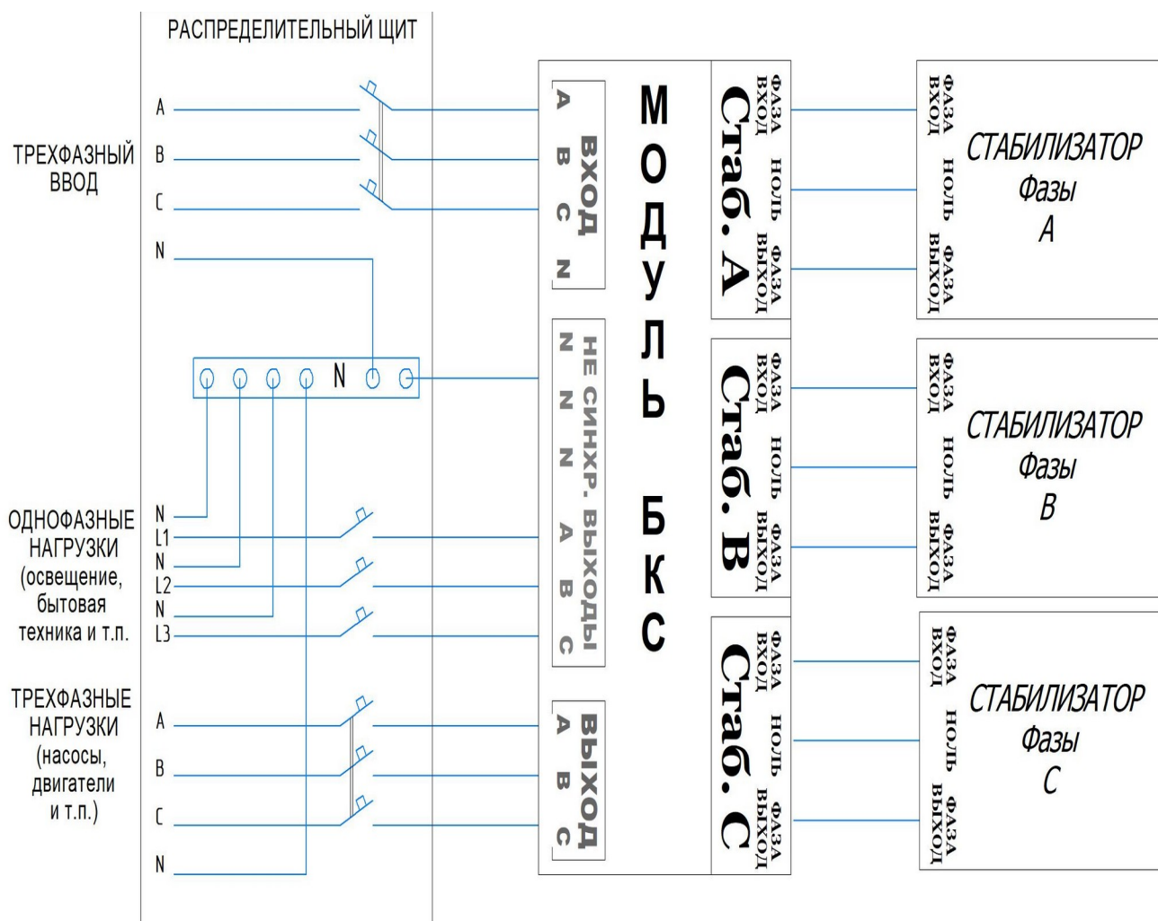
Рисунок 1. Рекомендуемая схема подключения Модуля БКС к сети.
